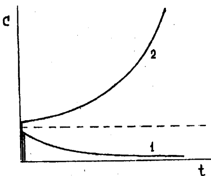
Рис. 2. Кинетика нарастания концентрации тромбина при подпороговой (1) и надпороговой (2) активации системы свертывания. Пунктиром показано пороговое значение активации [5].
