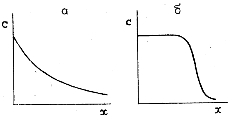
Рис. 1. Распределение концентрации вещества ( C ) вдоль пространственной координаты ( x ) при диффузионном ( a ) и автоволновом ( b ) распространении.
