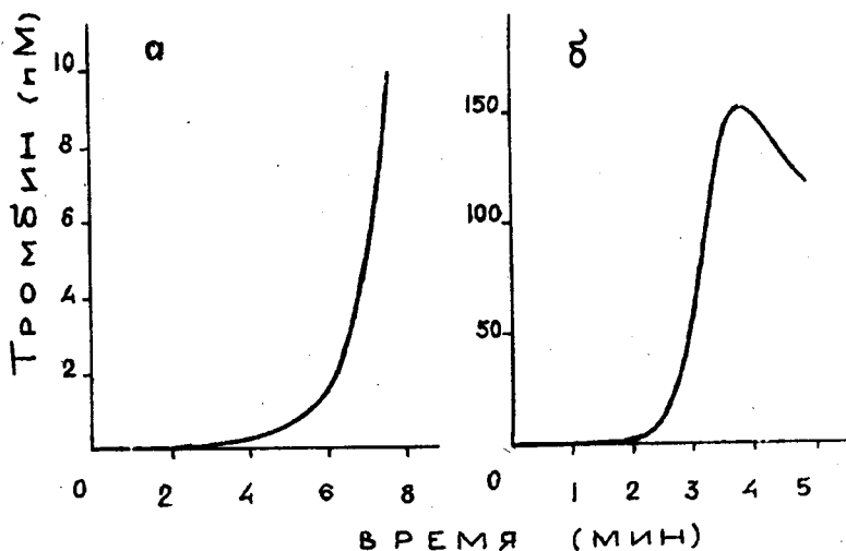
Рис. 3. Кинетика нарастания концентрации тромбина при активации внутреннего (а) [7] и внешнего (б) [8] путей системы свертывания.
